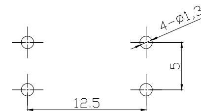
PCB. 焊接图
