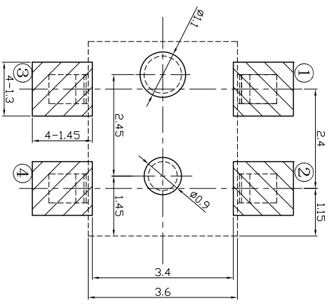
安装位置图
