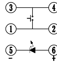
电原理图
