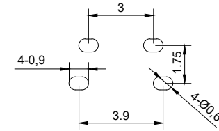
PCB. 焊接图
