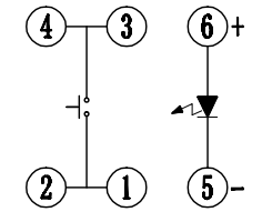
电原理图
