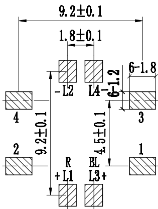
元件面孔位图
