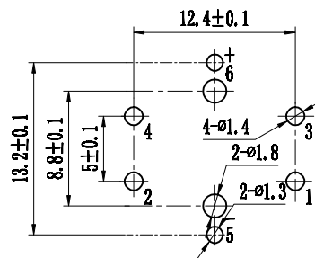
元件面孔位图
